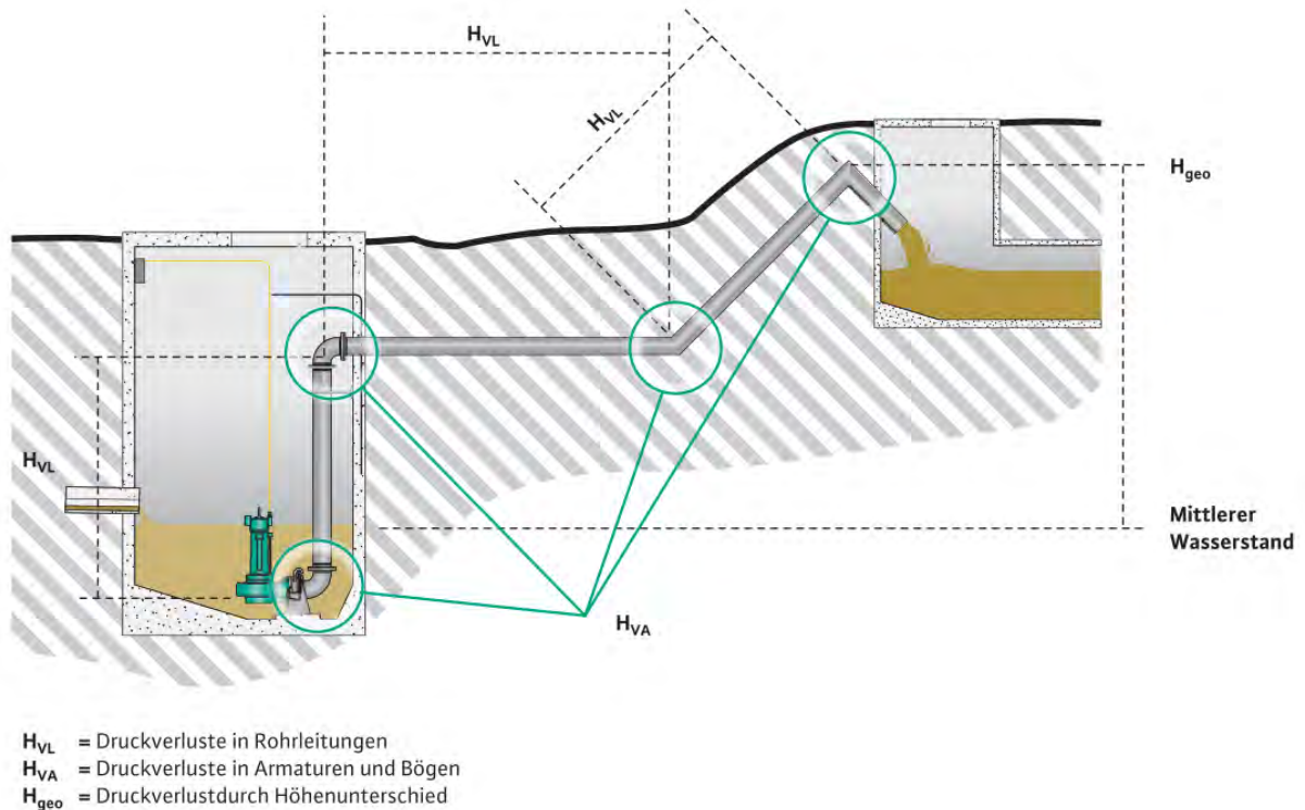
Abbildung 4-7: Anteile der Förderhöhe (WILO, 2008)
