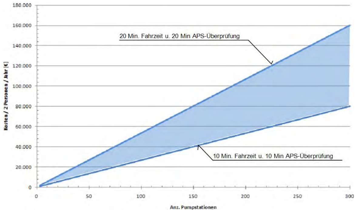
Abbildung 4-42: Jährliche Gesamtkosten in Abhängigkeit von der APS-Anzahl bei 10-maliger vor-Ort-Überprüfung pro Jahr (PLIHAL et al., 2011)
