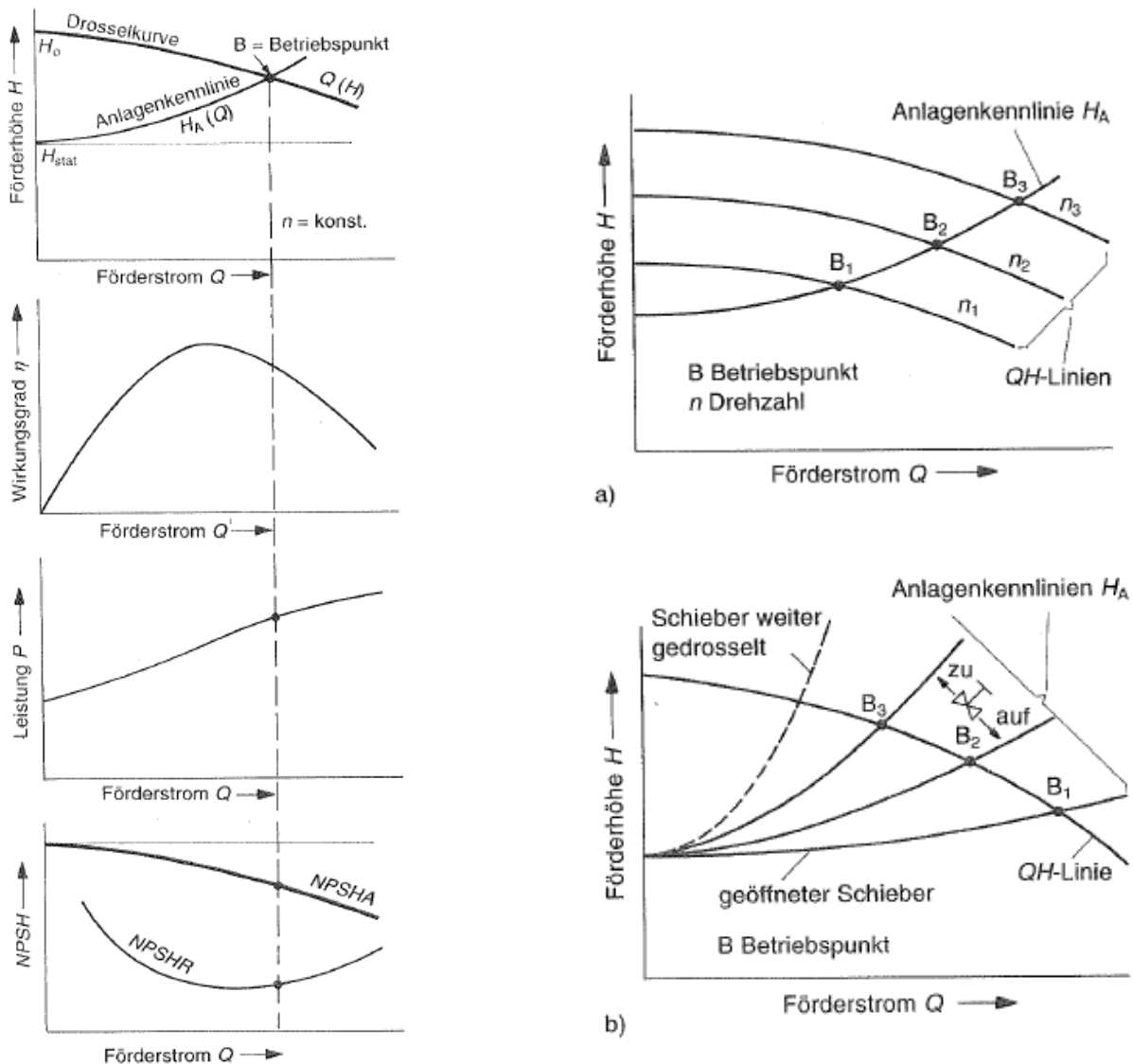
Abbildung 4-19: Ermittlung des Betriebspunktes (WAGNER, 1994)
