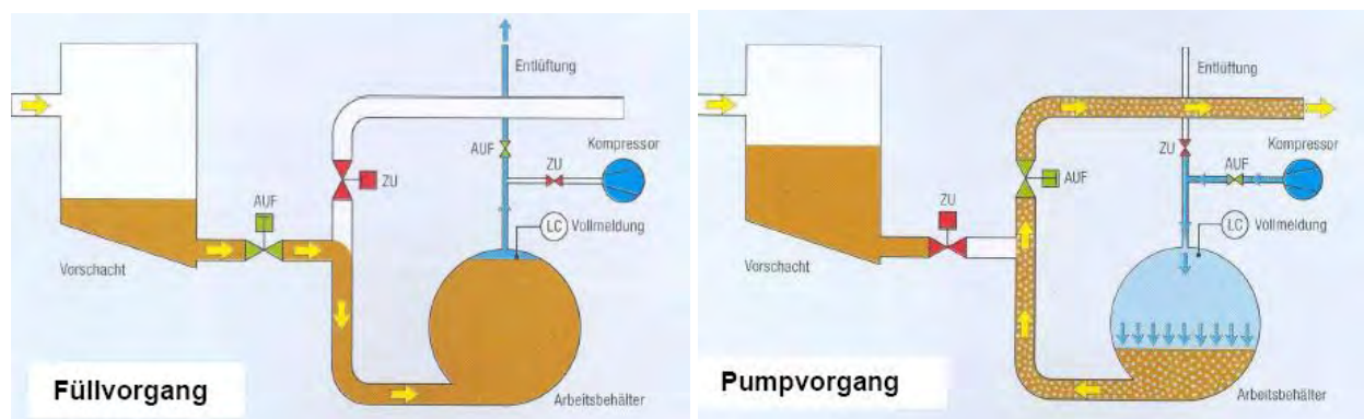
Abbildung 3-12: Funktionsschema einer pneumatischen Überdruckförderung System GULLIVER® (HOELSCHERTECHNIK, 2011)
