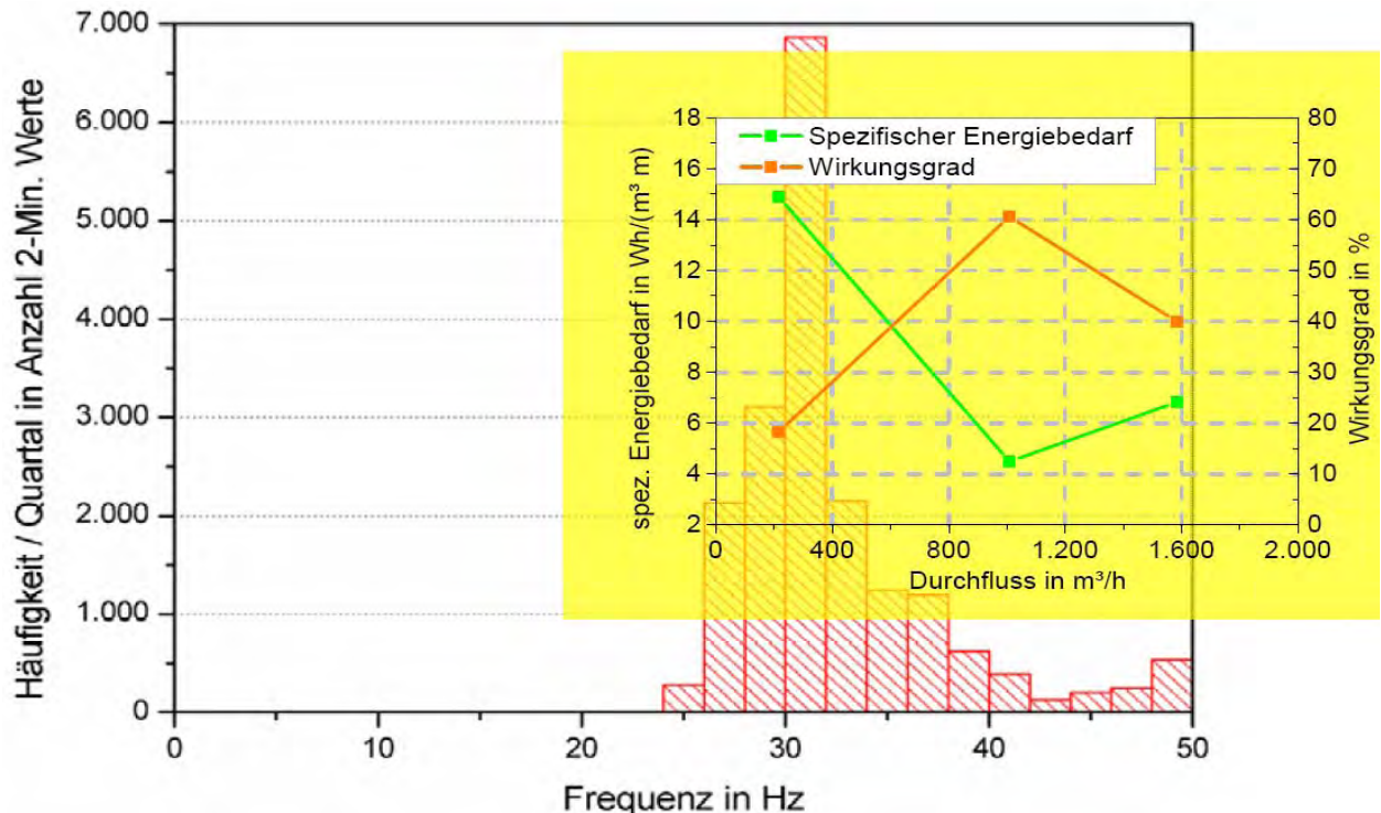
Abbildung 9-7 – Vergleich spezifischer Energiebedarf und Wirkungsgrad bei Abwasser-Pumpstationen (SEIBERT-ERLING, 2010a)
