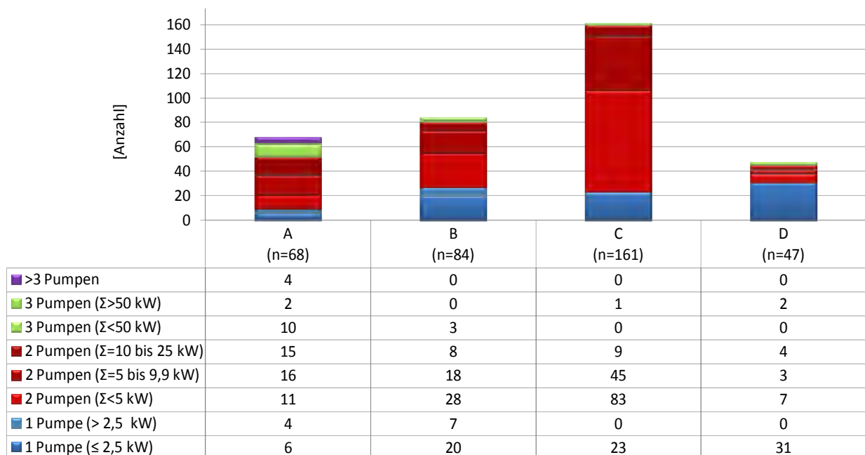
Abbildung 8-13: Aufteilung der PW in Anzahl Pumpen und installierter Pumpenleistung nach Betreiber
