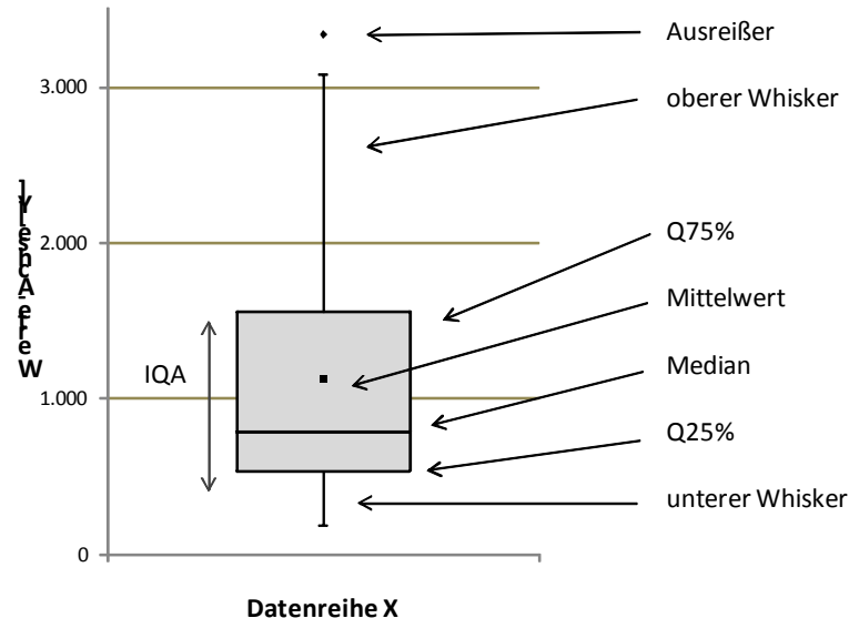
Abbildung 8-1: Boxplot-Darstellung
