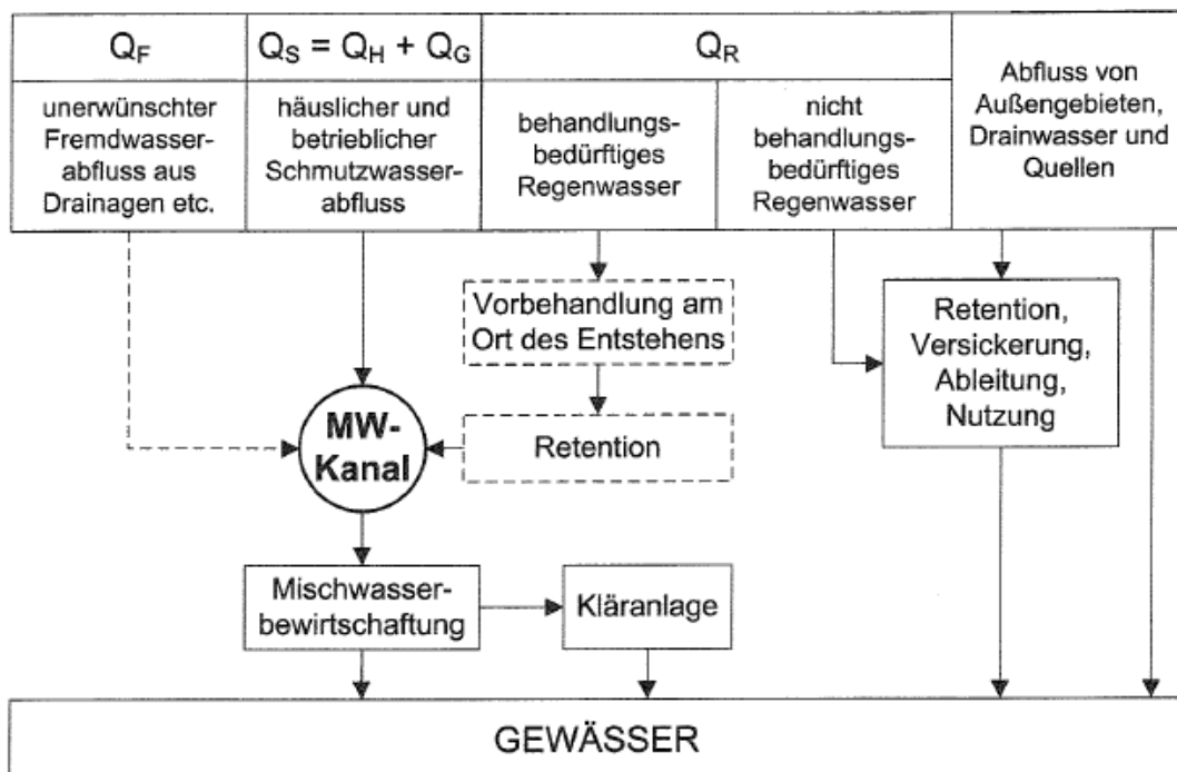
Abbildung 3-6: Schema modifiziertes Mischsystem (ÖWAV-Regelblatt 9, 2008)
