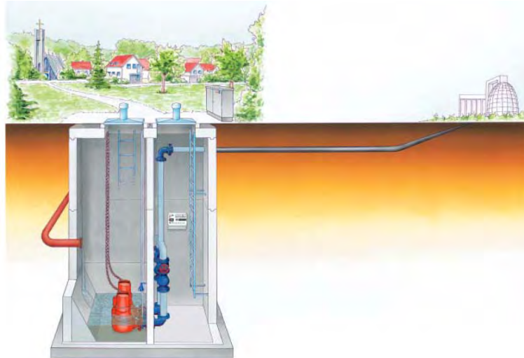
Abbildung 4-4: Pumpstation mit nassaufgestellten Pumpen und trocken aufgestellten Armaturen (KORDES, 2011)
