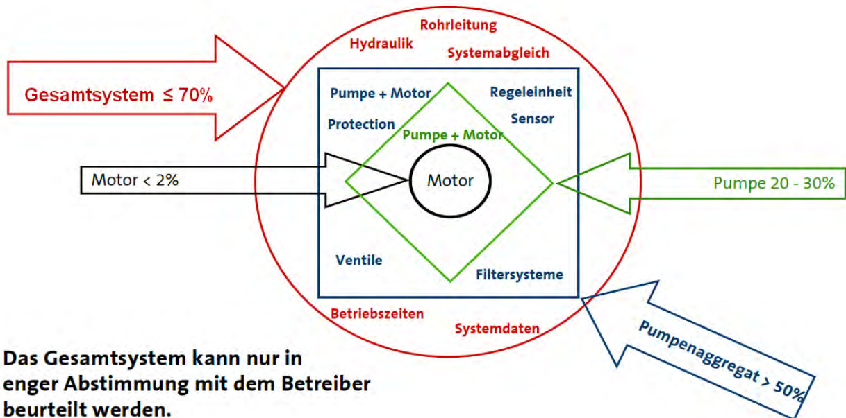
Abbildung 9-8 – Optimierung der Energieeffizienz (adaptiert nach SÖRENSEN, 2010)
