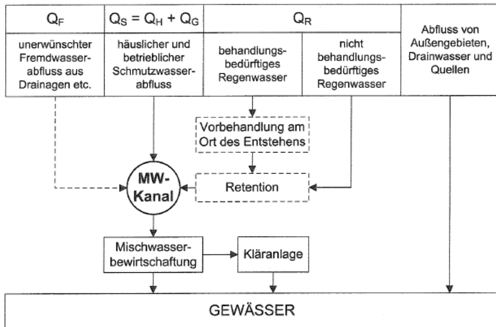
Abbildung 3-5: Schema Mischsystem (ÖWAV-Regelblatt 9, 2008)
