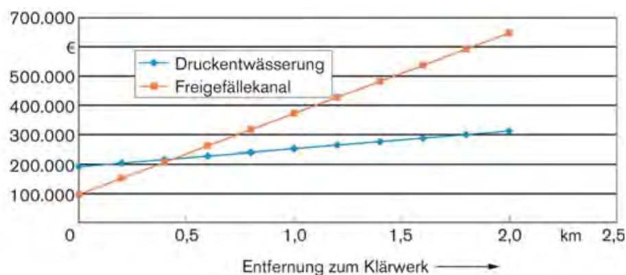
Abbildung 6-7: Investitionskostenvergleich Freigefällekanalisation vs. Druckentwässerung (KÄMPF, 2009)
