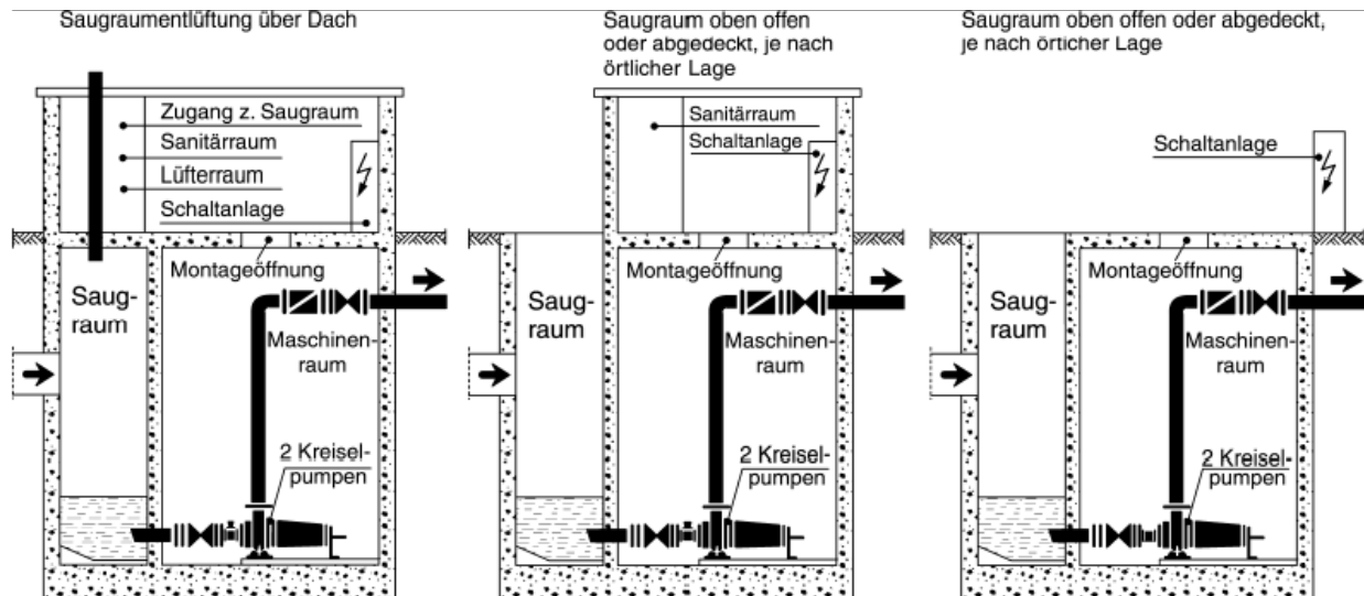
Abbildung 4-5: Beispiele für Pumpwerksbauarten mit Pumpen in Trockenaufstellung (ATV-DVWK-A134, 2000)
